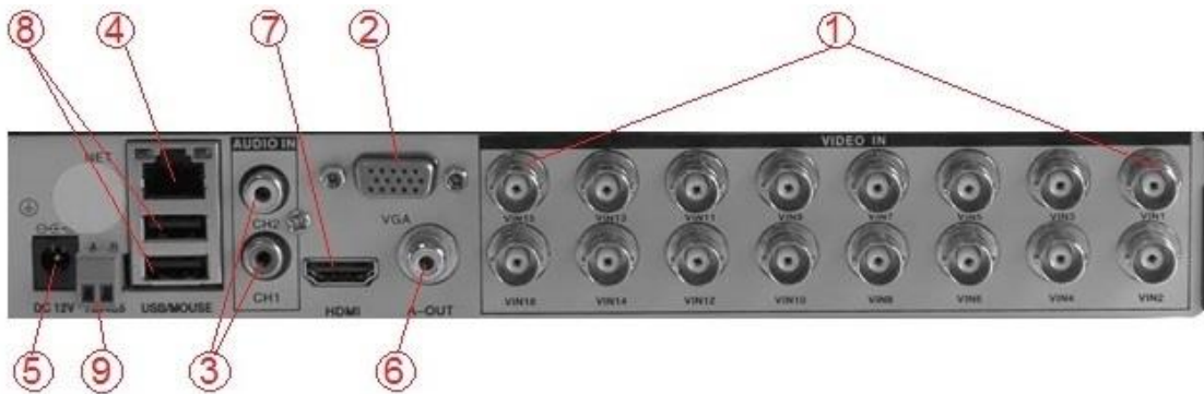
Задняя панель CTV-HD916A LITE
